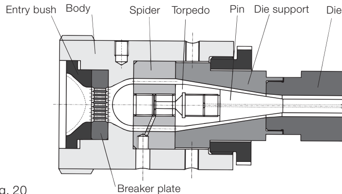
Tube extrusion die
